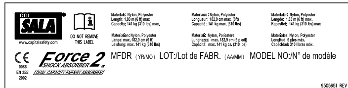
Especificaciones del material, Shockwave2 Force2 Modelos de energía eólica
