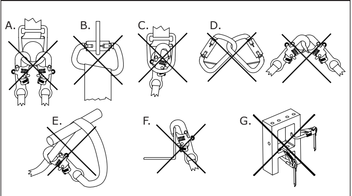
Figura 6 – Conexiones inapropiadas
