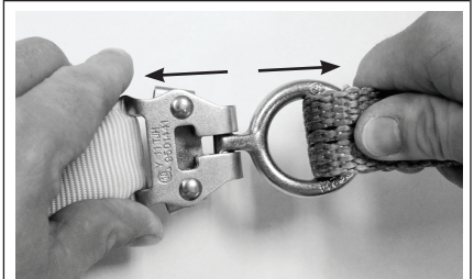
Figura 12 – Conexión fallida
